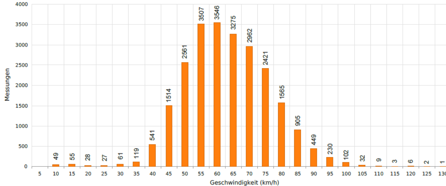
Zeckendorfer Straße, stadteinwärts , 50 km/h Beschränkung Anzahl der Messwerte vs. Geschwindigkeit
