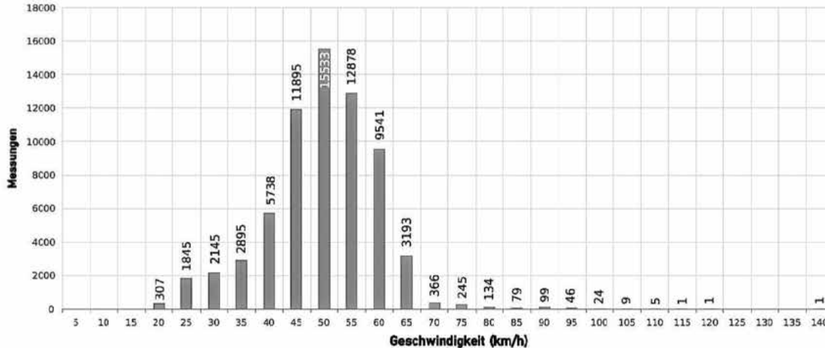
Giecher Straße, von Wiesengiech kommend zur Ortsmitte, 50 km/h Beschränkung Anzahl der Messwerte vs. Geschwindigkeit
