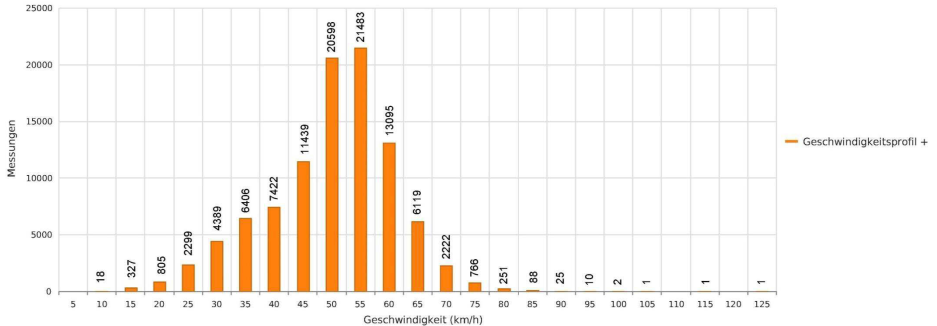
Oberend beim Pendlerparkplatz, Fahrtrichtung Stadtmitte, 50 km/h Beschränkung Anzahl der Messwerte vs. Geschwindigkeit
