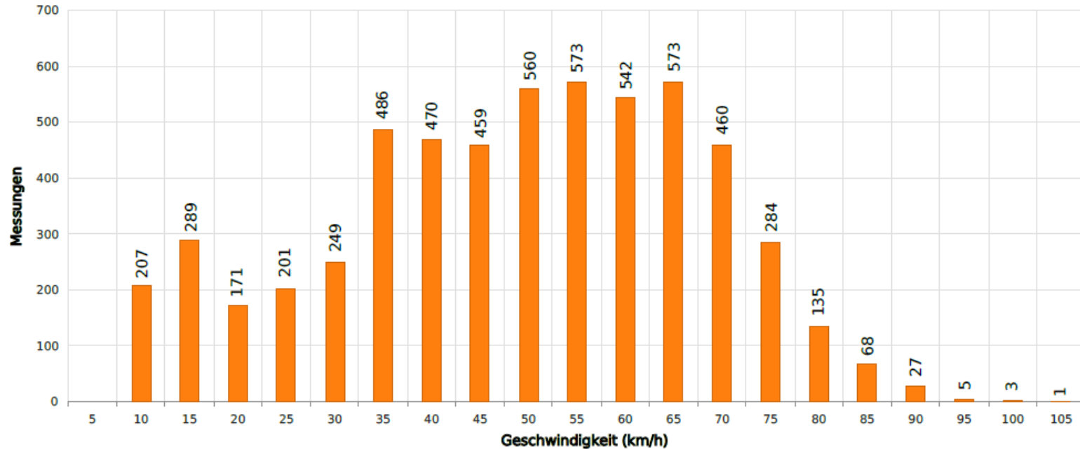
BA30, von Ludwag kommend zur Ortsmitte, 50 km/h Beschränkung Anzahl der Messwerte vs. Geschwindigkeit
