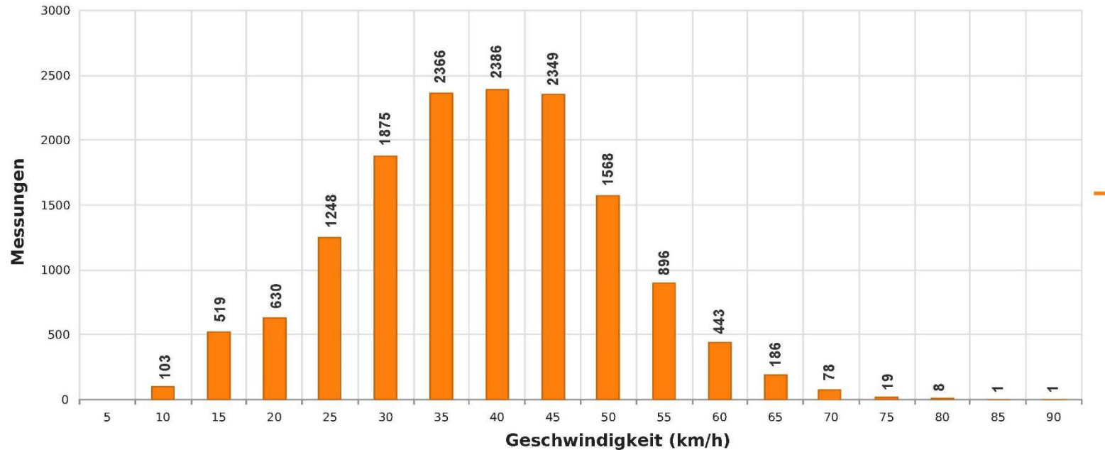
Schulstraße, in Fahrtrichtung Ortsmitte, Zone 30 Anzahl der Messwerte vs. Geschwindigkeit
